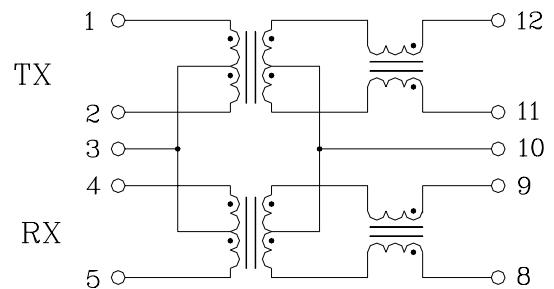
12PS6121UX
