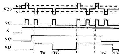
图4 可重复触发工作方式下各点的波形
