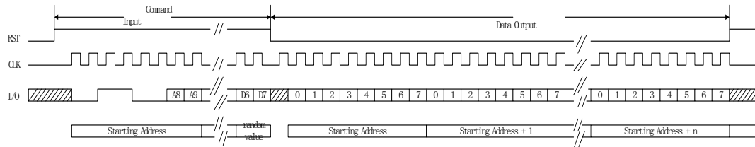
图 7 读数据字节时序
