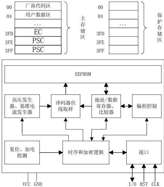
图 2 电路框图和存储空间分布
