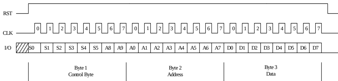
图 4 命令输入时序图
