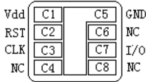
图 1 管脚图
