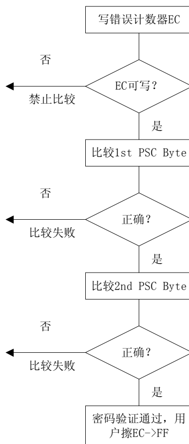
图 9 密码验证流程
