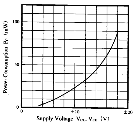
P_C - V_{CC}, V_{EE}
