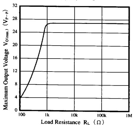
V_{O(max.)} - R_L
