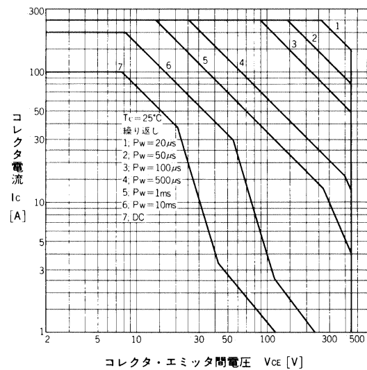
安全動作領域特性
