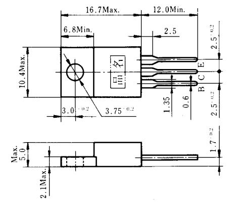
外形寸法 (単位: mm)
