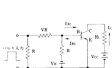
スイッチング特性測定回路
